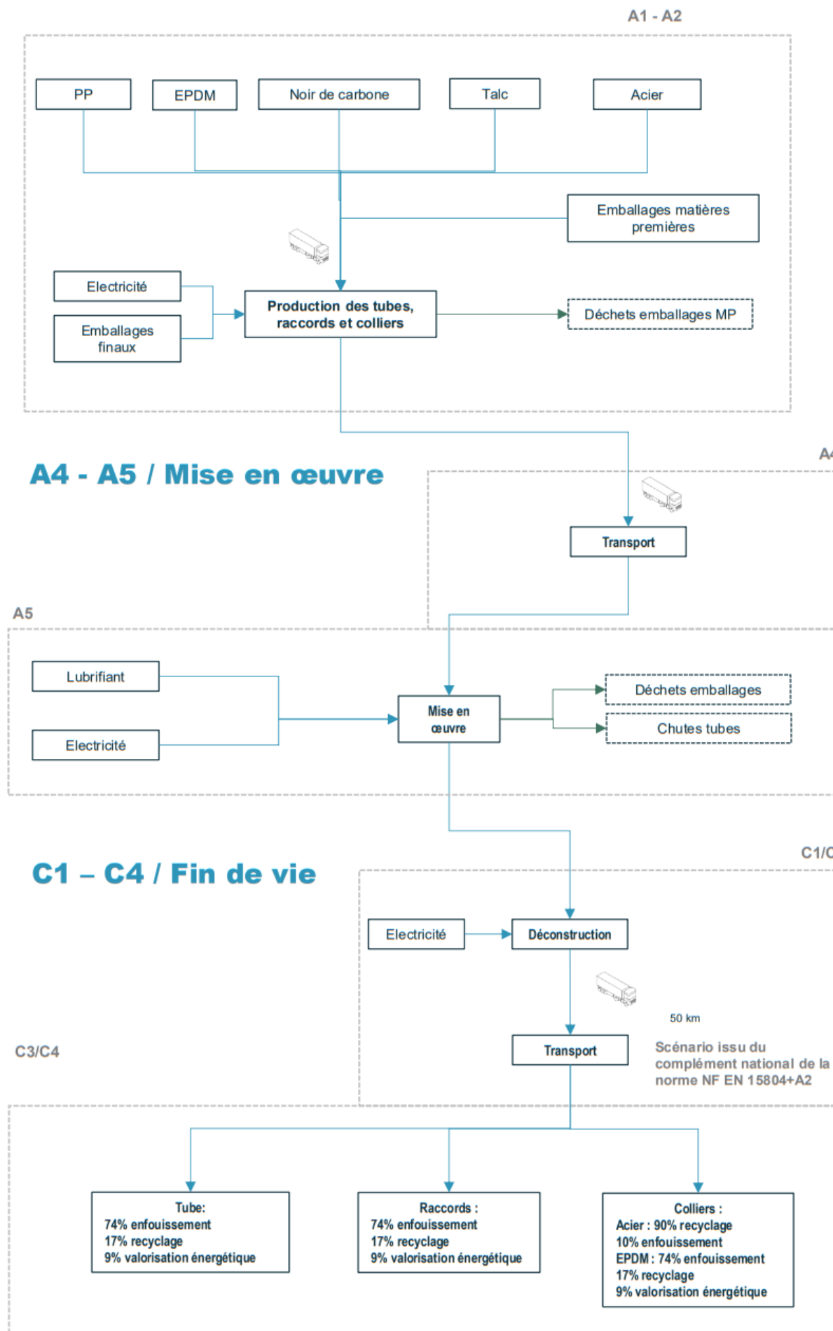
Diagramme de flux
